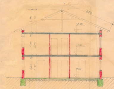
SCHNITT A-A
