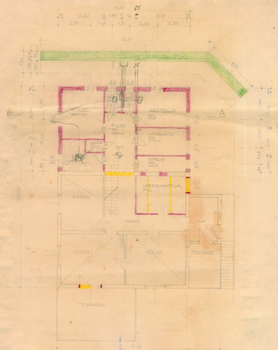
ERDGESCHOSS
