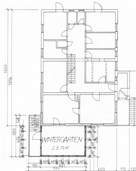
ERDGESCHOSS
